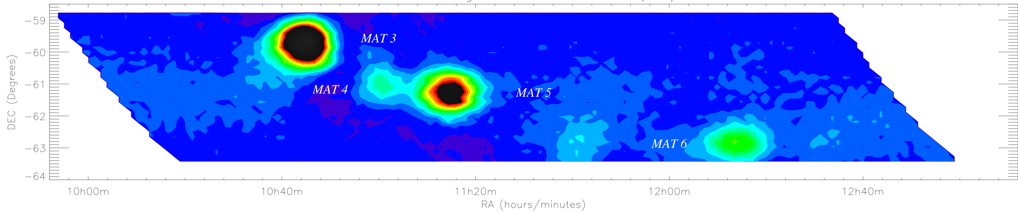
Galactic Region Observed at 30 GHz (Ka1)
